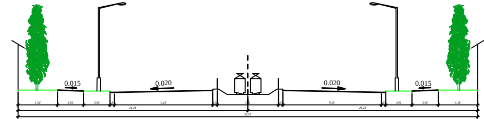
Поперечний профіль 1-1 просп. Леся Курбаса М1:200
