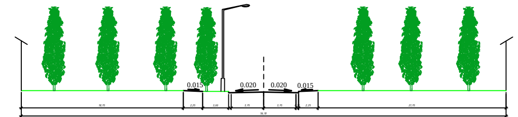
Поперечний профіль 2-2 просп. Академіка Корольова М1:200
