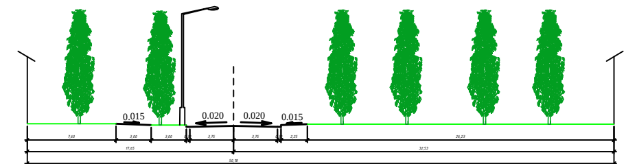
Поперечний профіль 3-3 вул. Героїв Космосу М1:200
